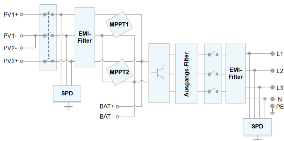
Abbildung 2-6 Konzeptdiagramm des SUN2000
